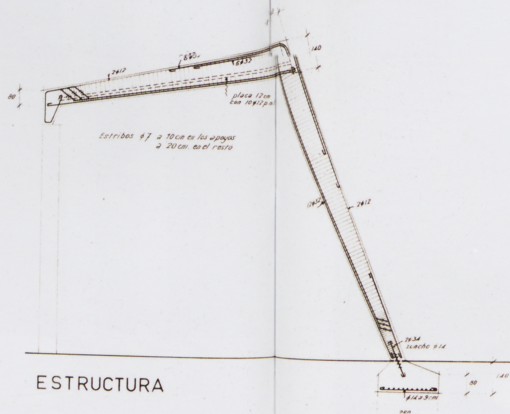
ALZADO DEL FONTIS
