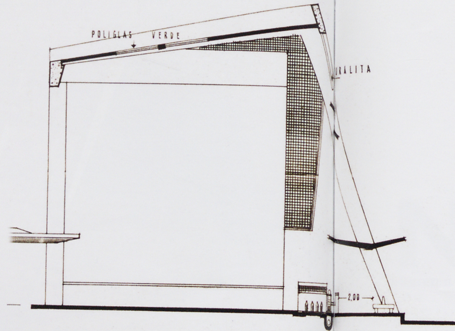
ALZADO DEL FONTIS
