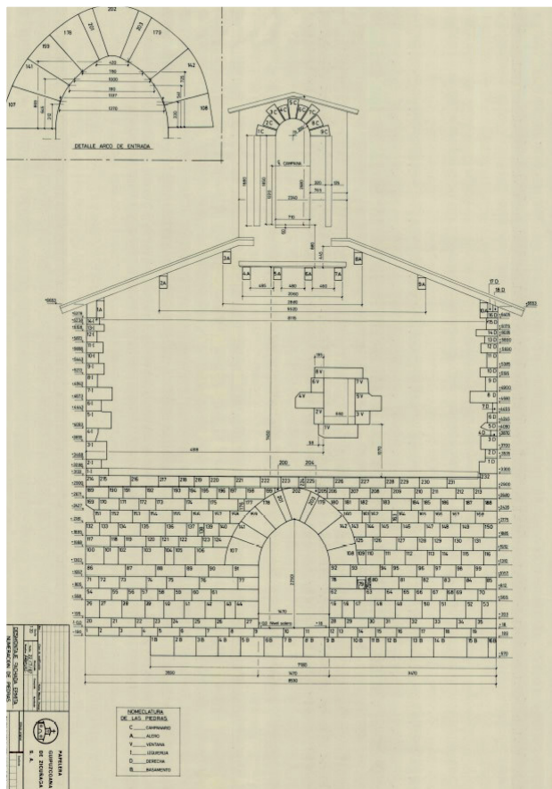
Plano de levantamiento de fachada, en el momento de su desmontaje (1987).
