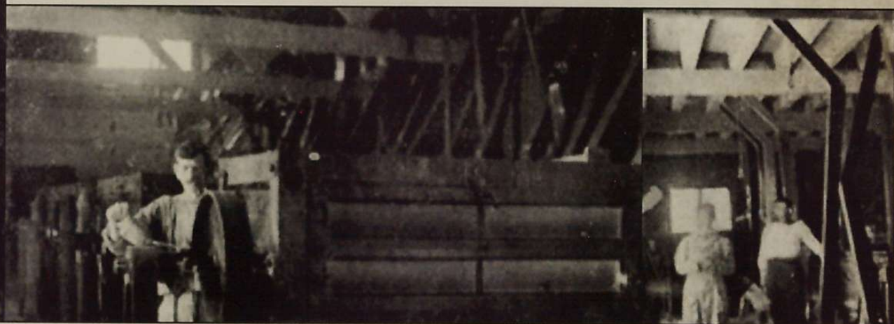
Elaboración por cilindros, produciendo diariamente 60.000 kilos de harina.
